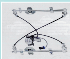
Стеклоподъемник для ВАЗ «Калина», «Гранта» под электропривод: передней левой двери, передней правой двери, задней левой двери, задней правой двери
