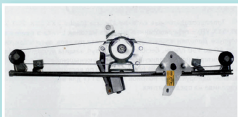
Стеклоподъемник для ВАЗ «Калина», «Гранта» под электропривод: передней левой двери, передней правой двери, задней левой двери, задней правой двери
